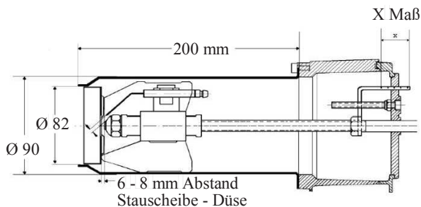
Stauscheiben
